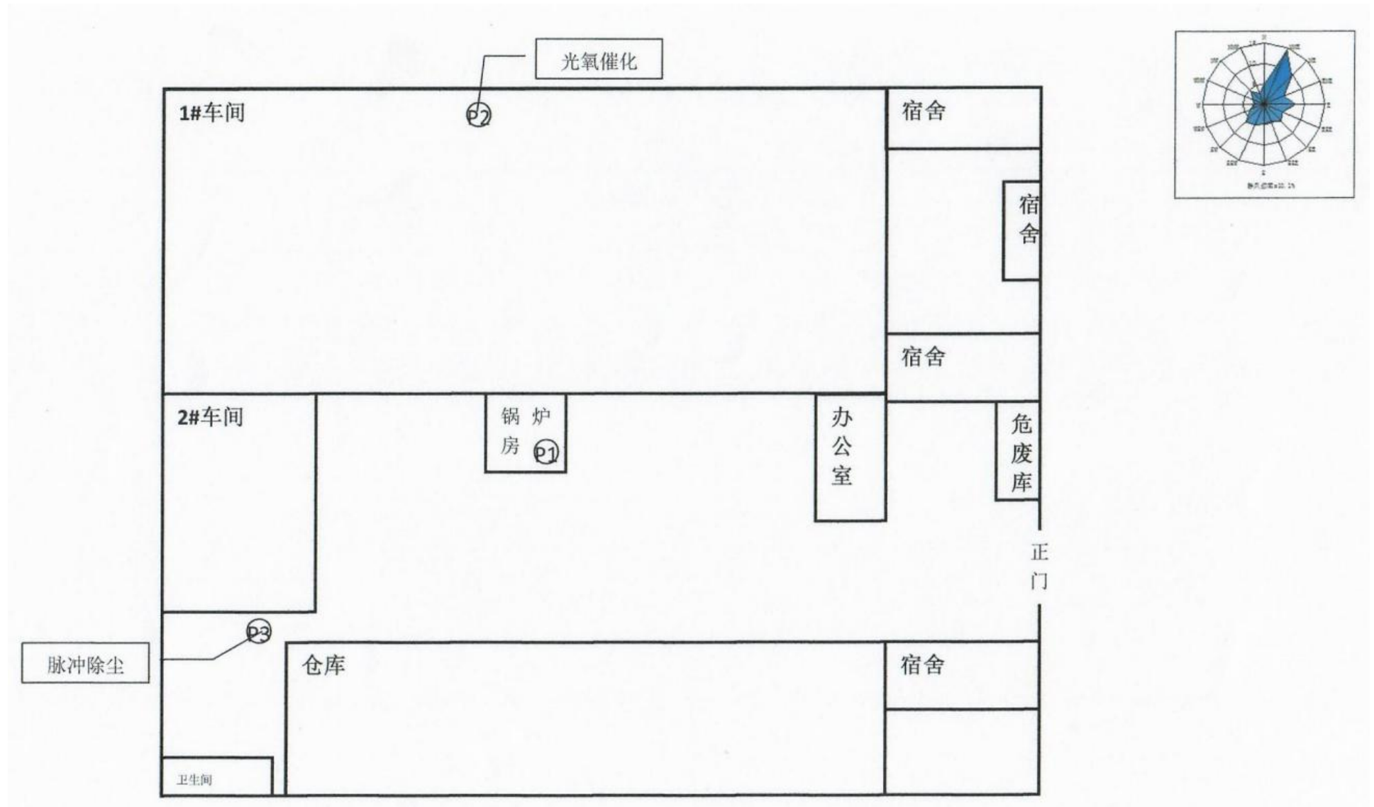
附图 3 本项目平面布置图
