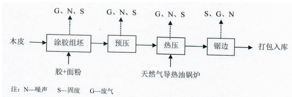
图 3-2 项目生产工艺流程及产污环节图
